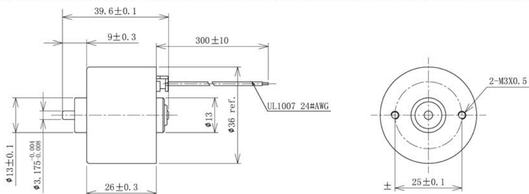
直流无刷电机 BLDC MOTOR
